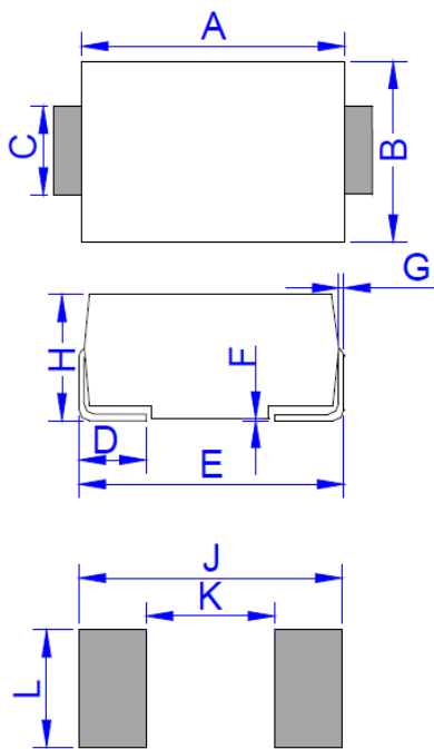
DO-214AB (SMC)
